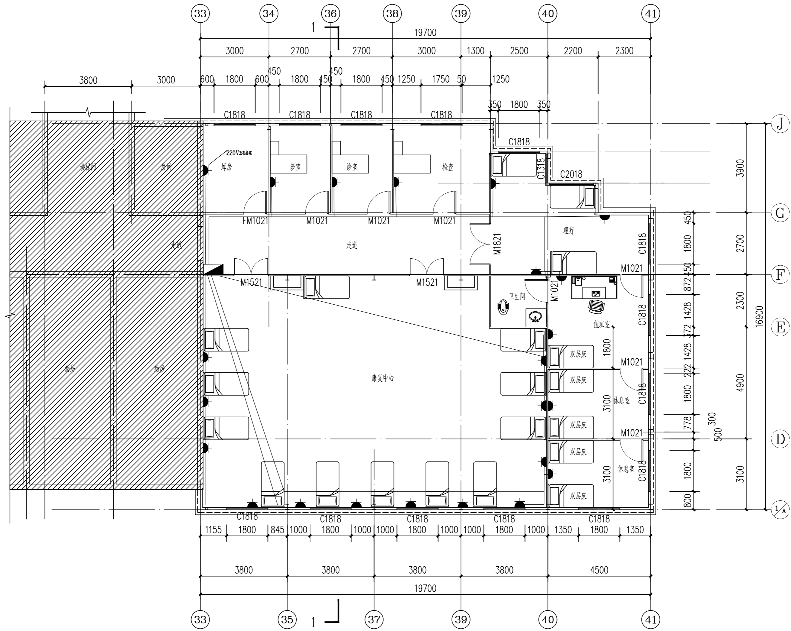
插座平面布置图 1:100
