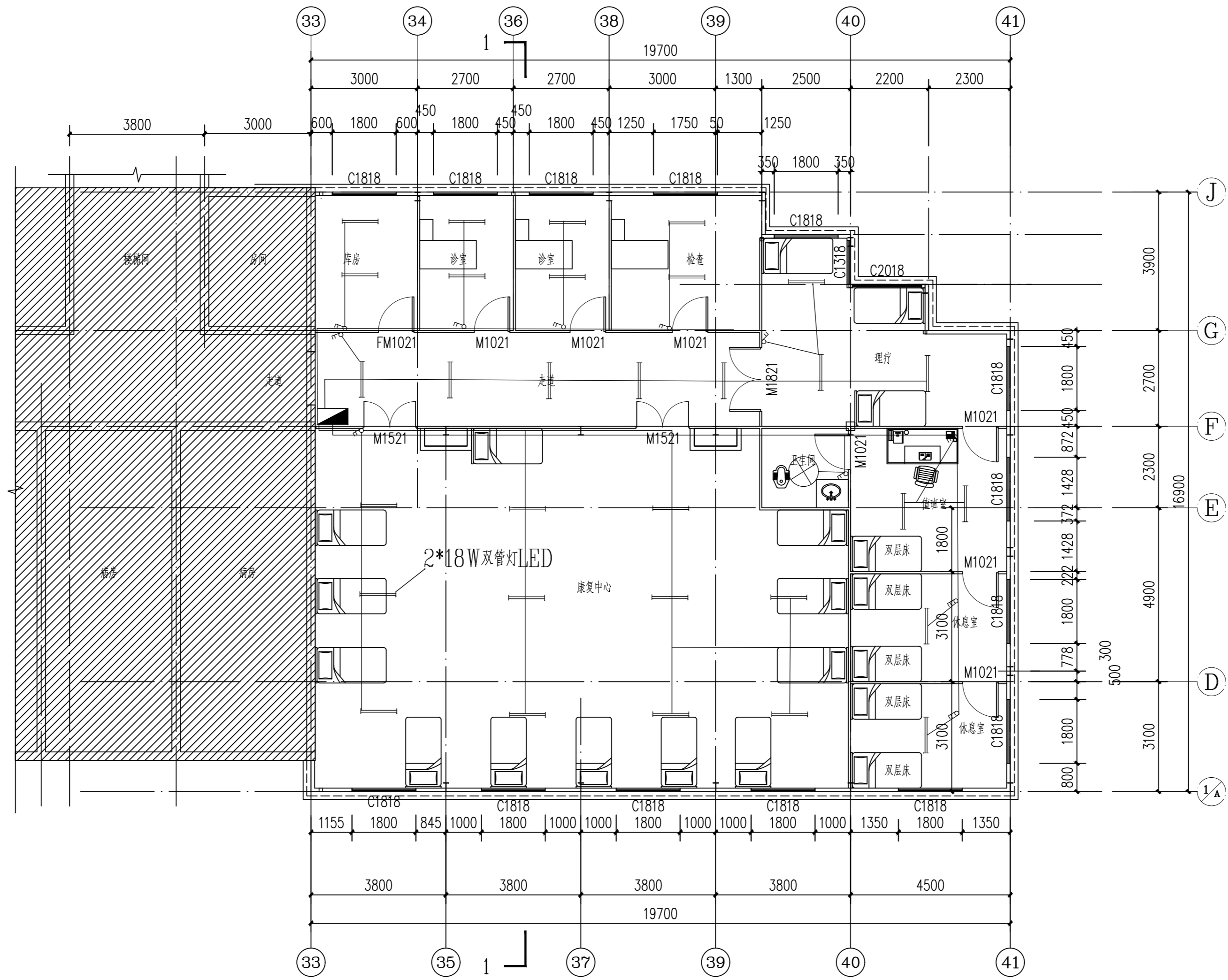
照明平面布置图 1:100
