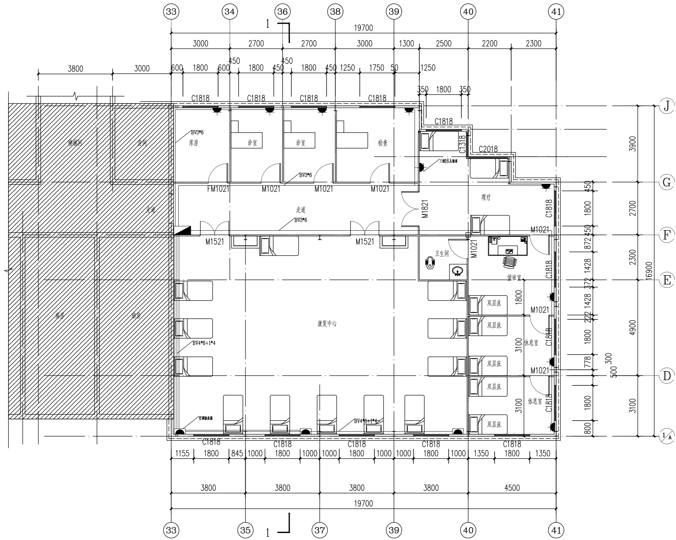
空调插座平面布置图
